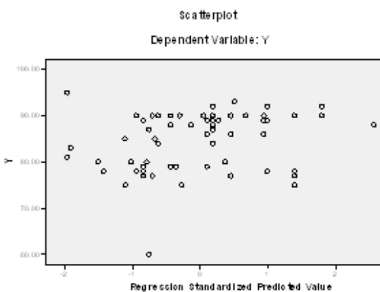
Gambar 2 Uji Heteroskedastisitas
